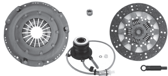
EJ-GM30HE 298mm (11 3/4") - 23.2 x 28.8mm / 10D Versión NO-Autoajustable
