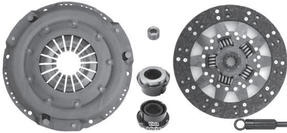
EJ-GM30FE 297mm (11 11/16") - 23.2 x 28.8mm / 10D Versión NO-Autoajustable
