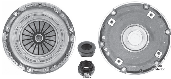
EJ-D24A Modular - Volante doble masa
